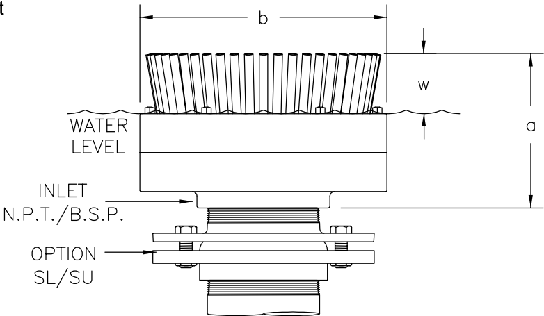
NSJ200 THRU 600
